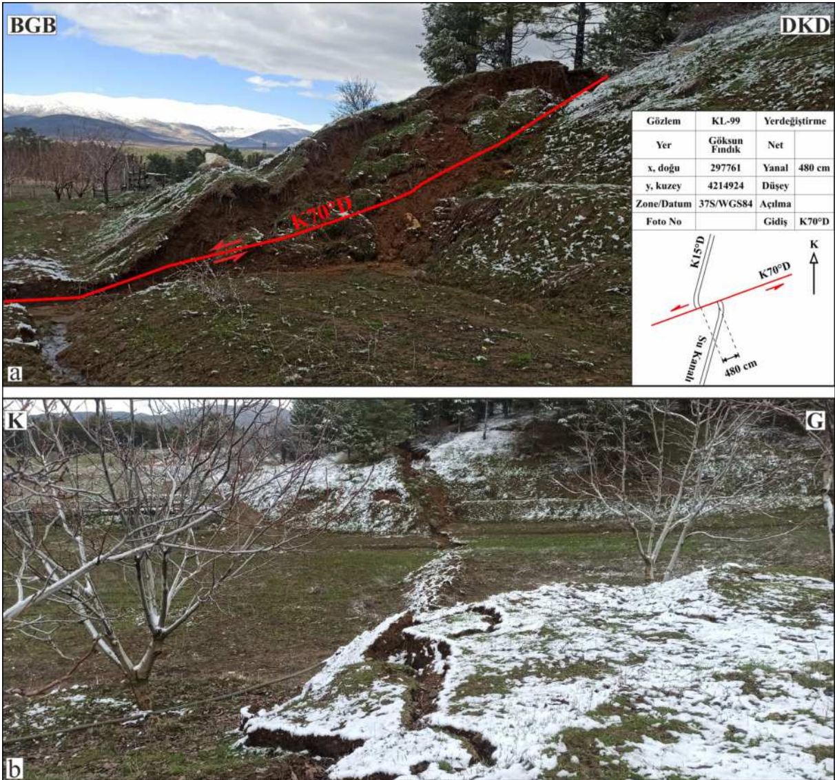
Şekil 8- Göksun İlçesi Gücüksü Köyü KD'sundaki a) yanall ötelenme (480±20 cm) ve b) yüzey kırığı boyunca gelişen köstebek izi yapısı.
