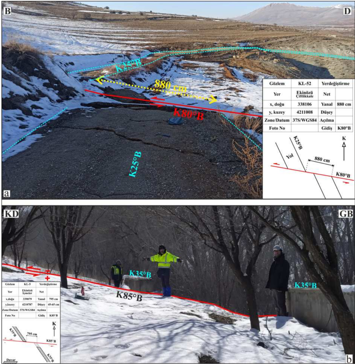
Şekil 9- a) Ekinözü İlçesi Aşağıçelmeler Köyü GB'sında bulunan yoldaki yer değiştirme (880±20 cm) ve b) Ekinözü İlçesi Aşağıçelmeler Köyü'ndeki yüzey kırığı ve bahçe duvarındaki yer değiştirme (795±5 cm).
