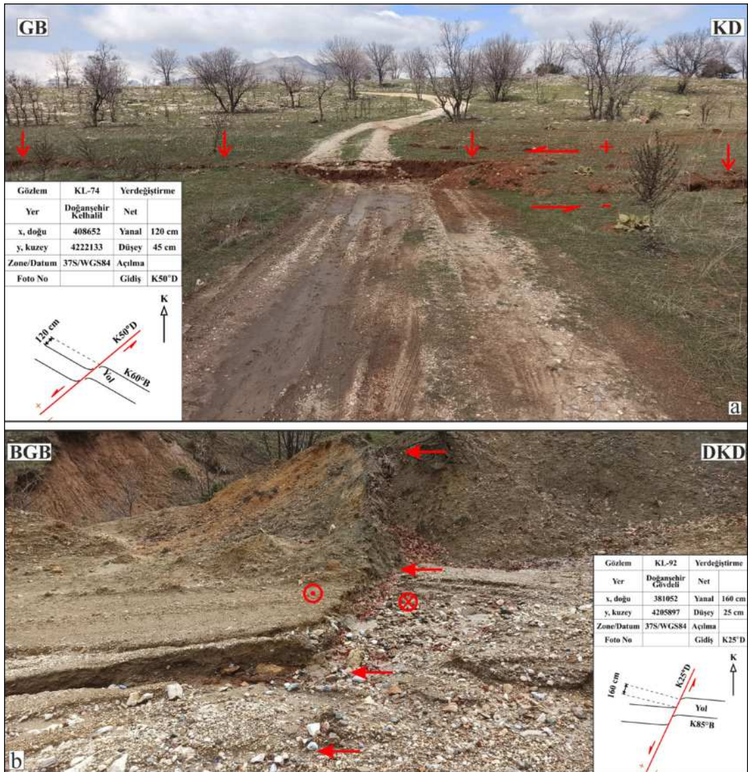
Şekil 14- a) Malatya ili Doğanşehir İlçesi Polatdere Köyü GD'sundaki yüzey kırığı ve yoldaki ötelenme (yanal ötelenme 120 \pm 15 , düşey ötelenme 45 \pm 5 cm) ve b) Bıçakçı Köyü'ndeki yüzey kırığı ve yoldaki ötelenme (yanal ötelenme 160 \pm 20 , düşey ötelenme 25 \pm 5 cm).
