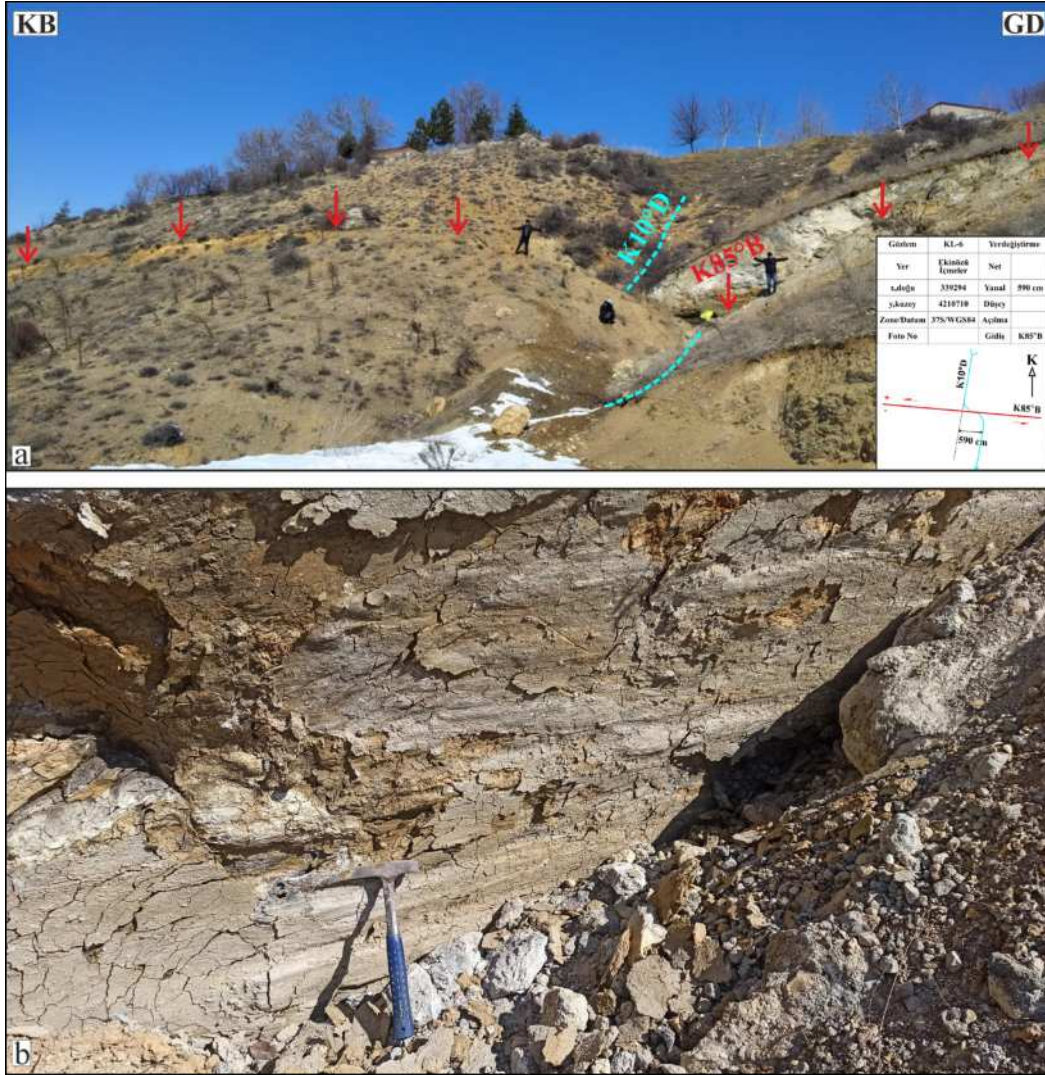
Şekil 10- Ekinözü İlçesi Aşağııçmeler Köyü'nde a) dere yatağındaki ötelenme ve kapatan sırt oluşumu (yanal ötelenme 590±20 cm) ve b) depremde oluşmuş fay yüzeyinin ve kayma çiziklerinin yakından görünümü.
