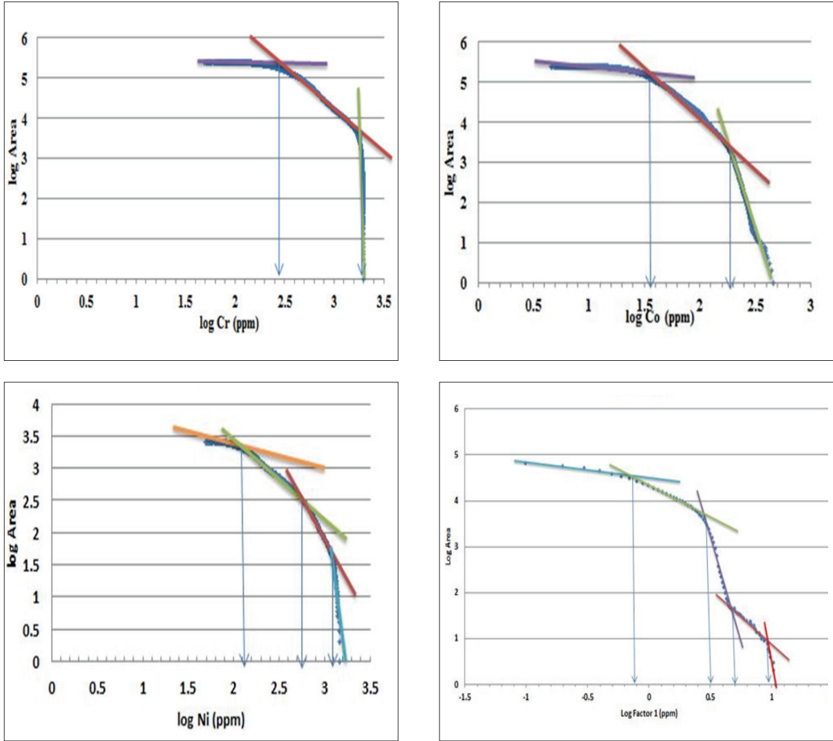
Şekil 4- Khoy paftasında Cr, Co, Ni ve Faktör 1 için C-A log-log grafiği.
