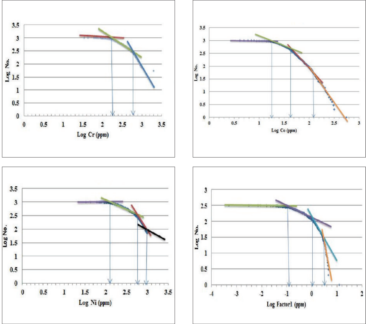
Şekil 3- Khoysaftasında Cr, Co ve Ni elementlerinin C-N log-log grafikleri.
