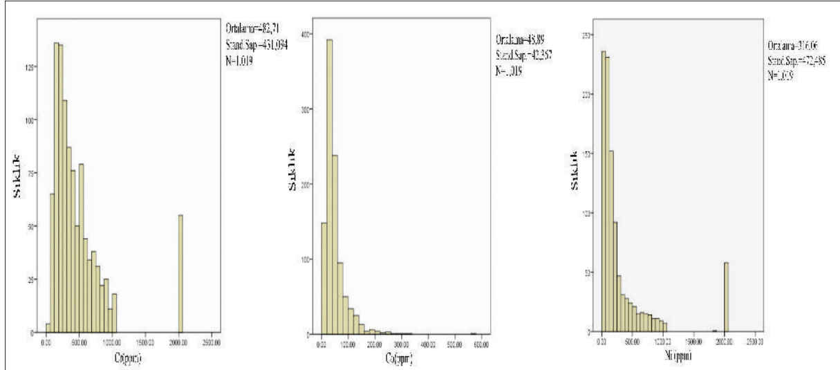
Şekil 2- Çalışma alanında Cr, Co ve Ni'in histogramları.
