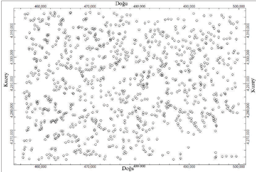
Şekil 1- Khoy 1:100.000 ölçekli paftanın jeolojisi ve İran'ın jeolojisi içinde yeri (Alavi, 1994'ten); bu alanda kalan kromit oluşukları ve dere sedimanı jeokimya örnek yerleri.
