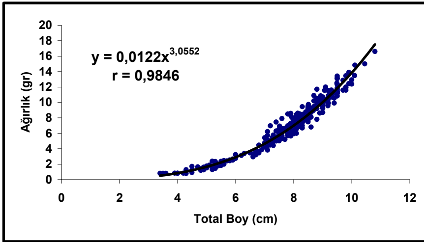
Şekil 3. L. klunzingeri bireylerinin total boy-ağırlık ilişkisi. Figure 3. Weight-length relationship of L. klunzingeri samples.
