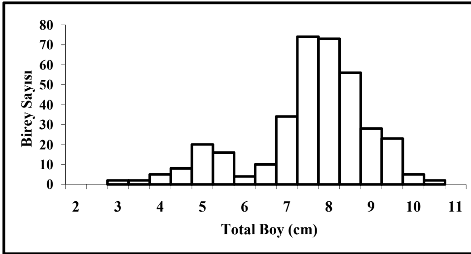
Şekil 2. L. klunzingeri bireylerinin boy frekans dağılımı Figure 2. Length frequency distribution of L. klunzingeri samples.
