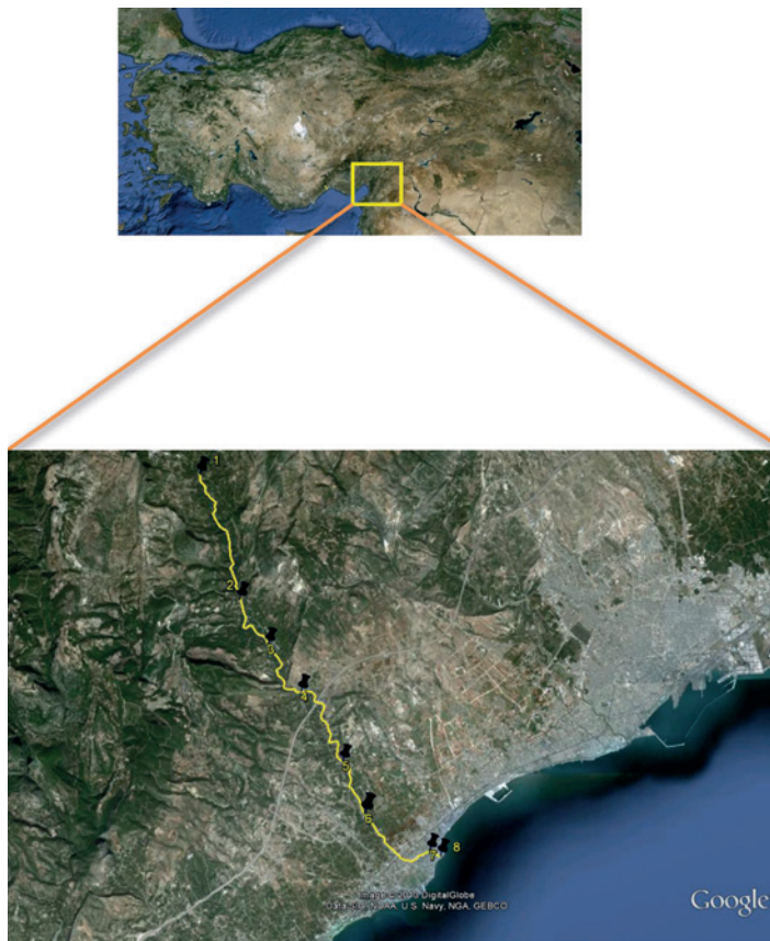
Şekil 1. Çalışma bölgesinin yer bulduru haritası.
