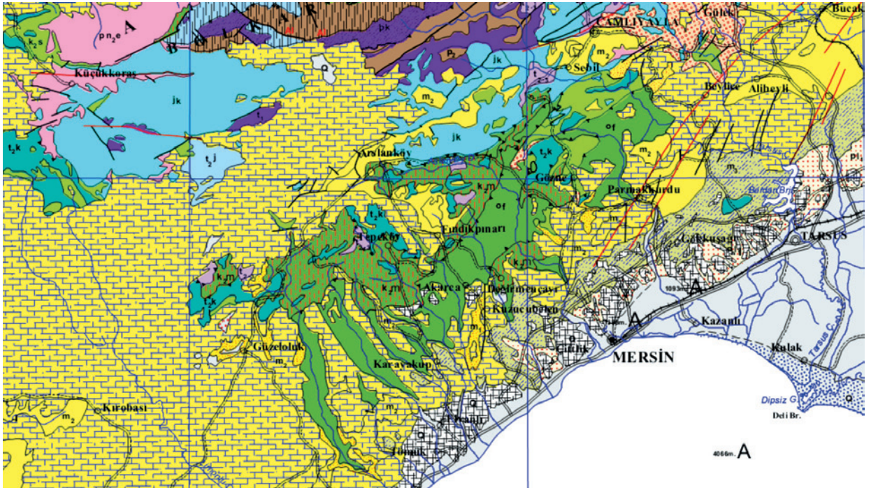
Şekil 2. İnceleme alanının jeoloji haritası (Şenol ve Duman 1998'den değiştirilerek).
