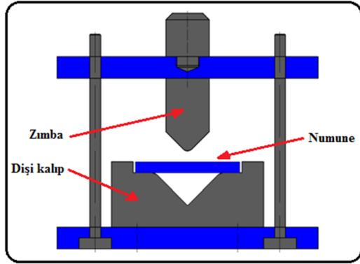
Şekil 2. Deneyisel çalışmalarda kullanılan bükme kalıbı
