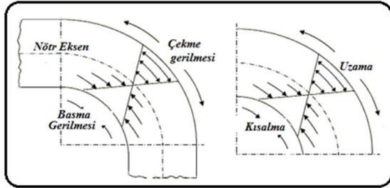
Şekil 1. Bükme işlemi neticesinde meydana gelen basma ve çekme gerilmesi (Compressive and tensile stresses occurring during the bending process)
