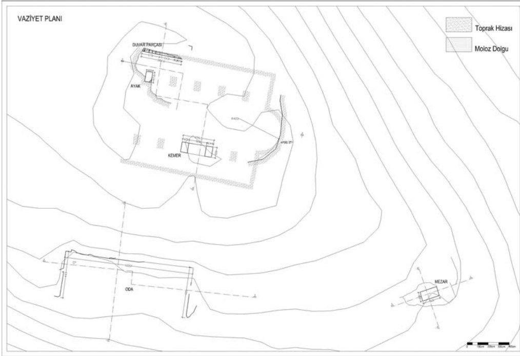
Res. 5: Zenonopolis Kilisesi, plan restitüsyonu.
