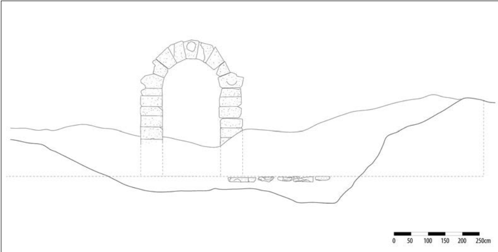
Res. 10: Zenonopolis Kilisesi, doğu-batı doğrultusunda geçen kesit, güneye bakış. Zeminde kaplama levhaları görülmektedir.
