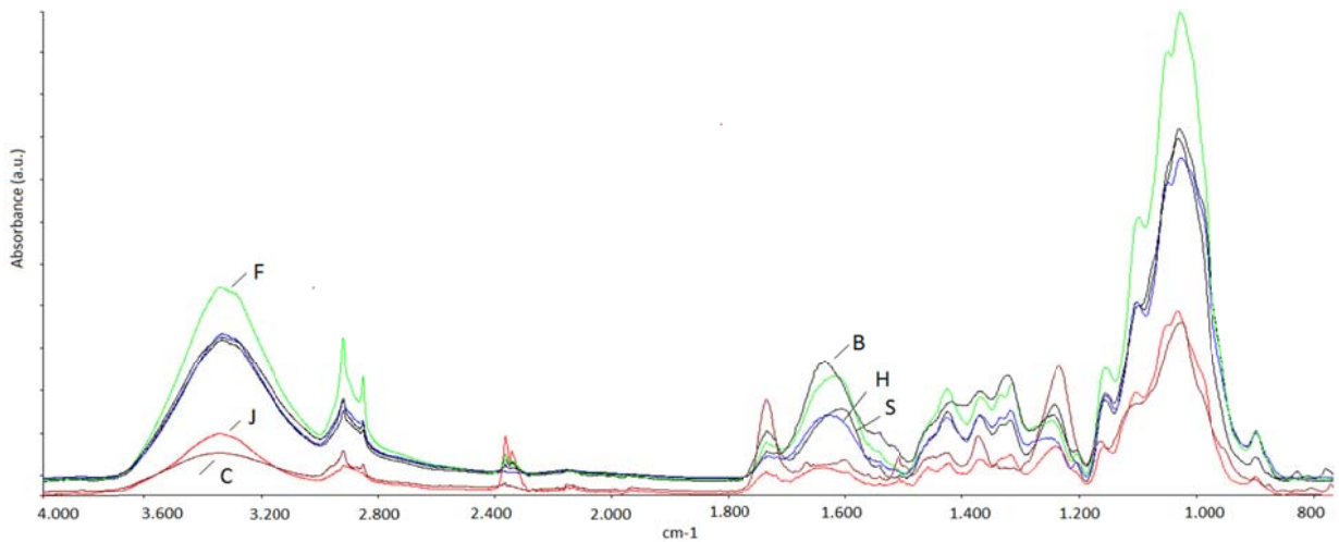
Şekil 2. Ham selülozik liflerin FTIR spektrumları
