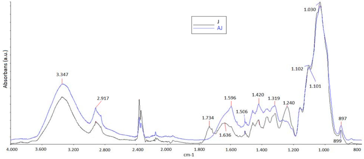
Şekil 8. Ham ve alkali ile modifiye edilen jüt liflerinin FTIR spektrumları (J:Ham jüt lifleri; AJ:Alkali ile modifiye jüt lifleri)
