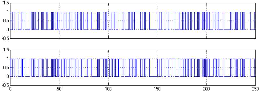
Şekil 13. a) İletilen bilgi sinyali b) Sproot FPGA alıcıda elde edilen bilgi sinyali.
